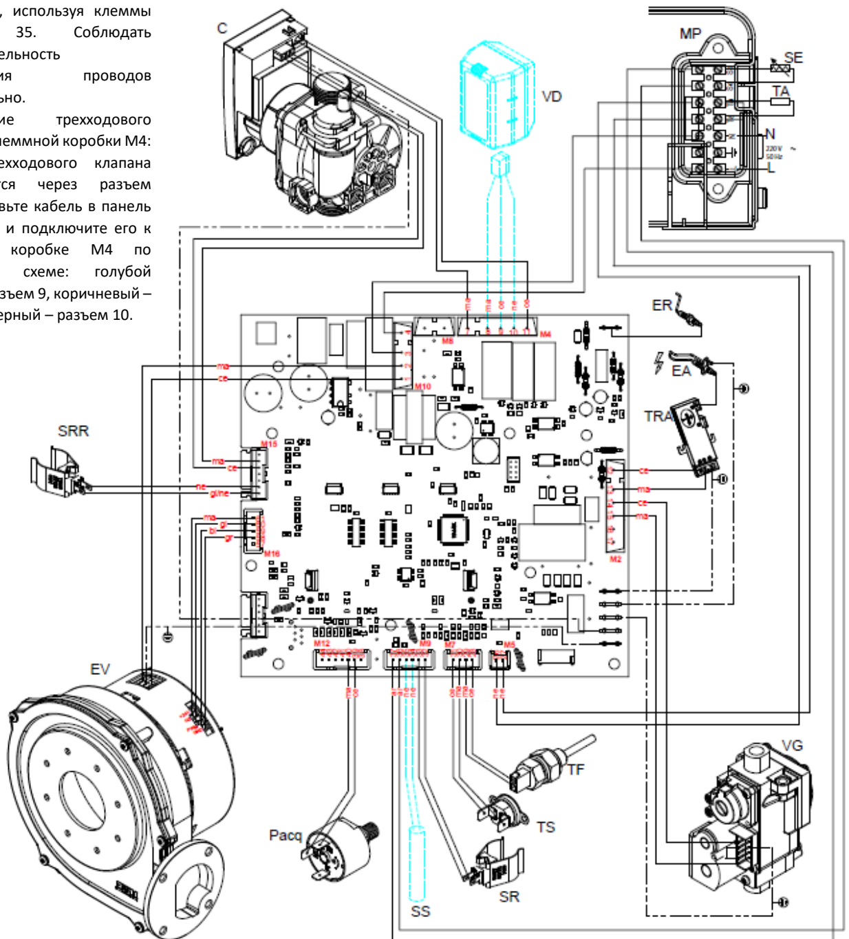
2. Электрическая схема_RU
